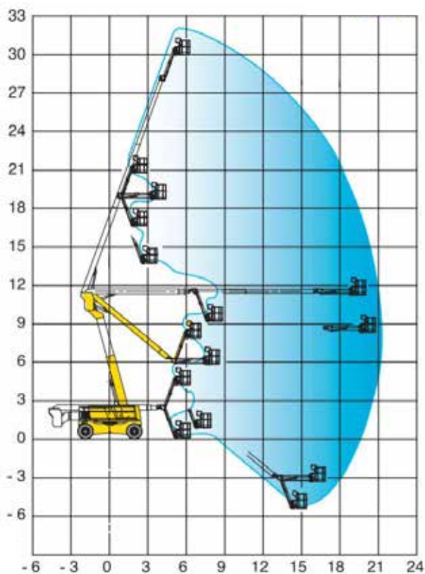
HAULOTTE HA32
